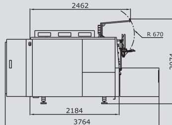
Seitenansicht
