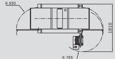
Draufsicht
